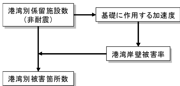
図5.3.1 揺れによる港湾施設の被害予測手順
