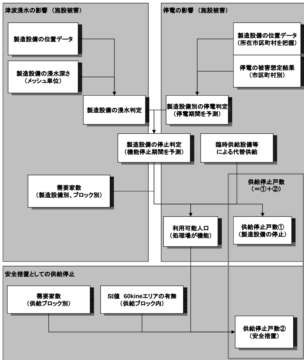
図4.5.1 都市ガスの供給停止戸数の想定フロー（内閣府（2013） [1] に基づく）
