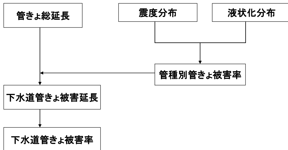
図4.2.2 下水道管きょ被害の予測フロー
