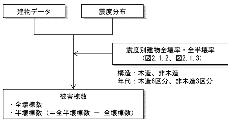
図2.2.1 揺れによる建物被害の想定フロー
