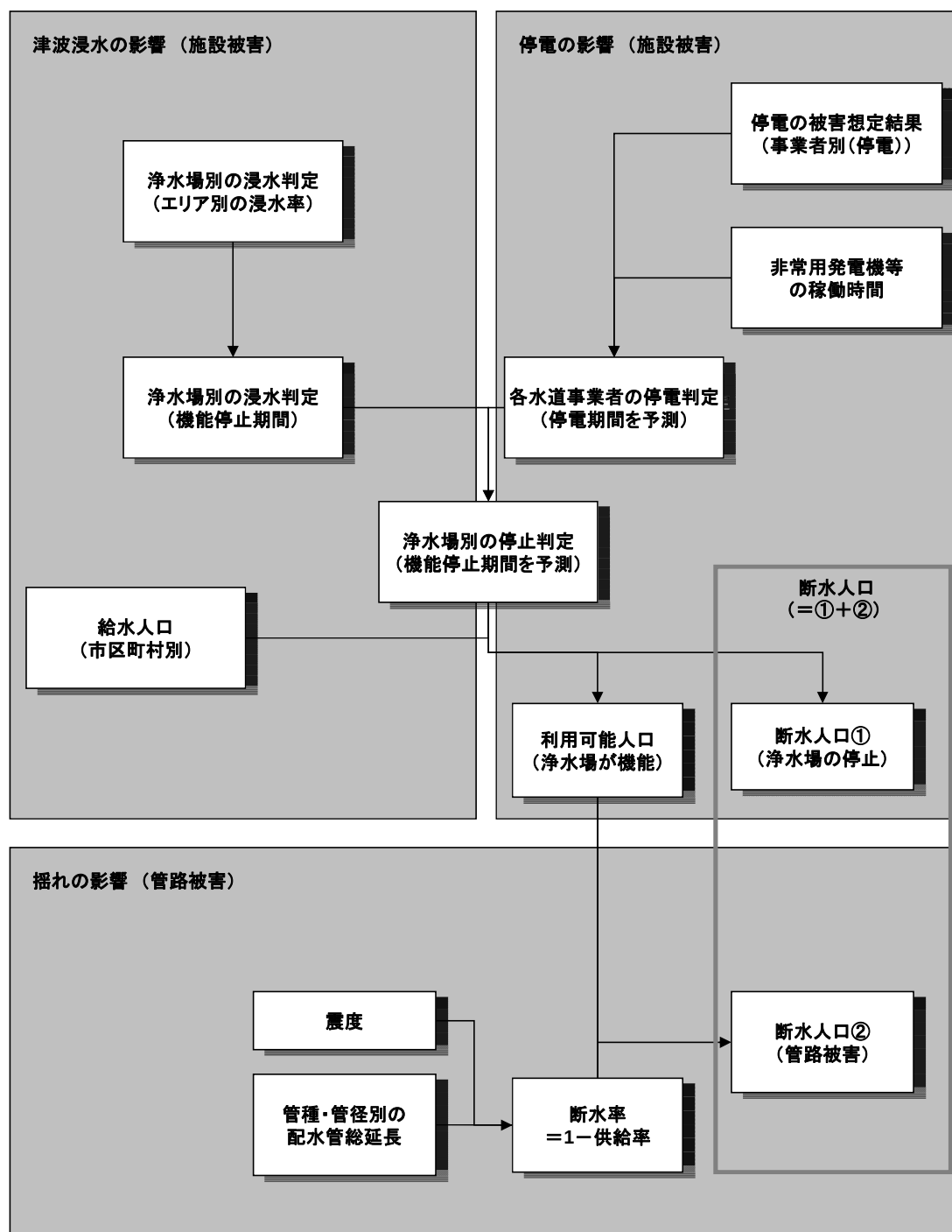
図4.1.1 上水道被害推定の全体フロー
