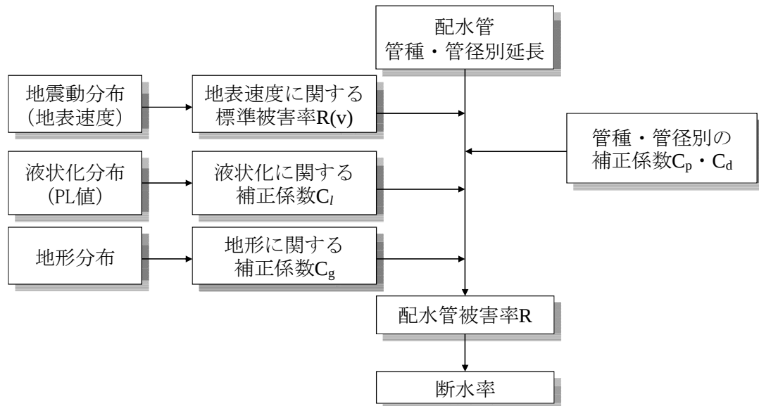
図4.1.2 上水道の管路被害の予測フロー
