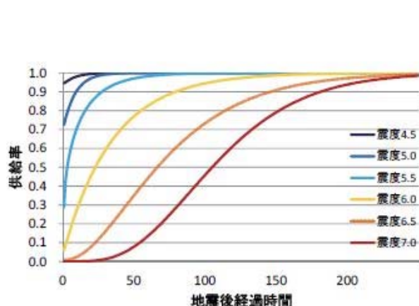
図 4.3.2 能島らによる震度と電力復旧推移の関係 [5]
