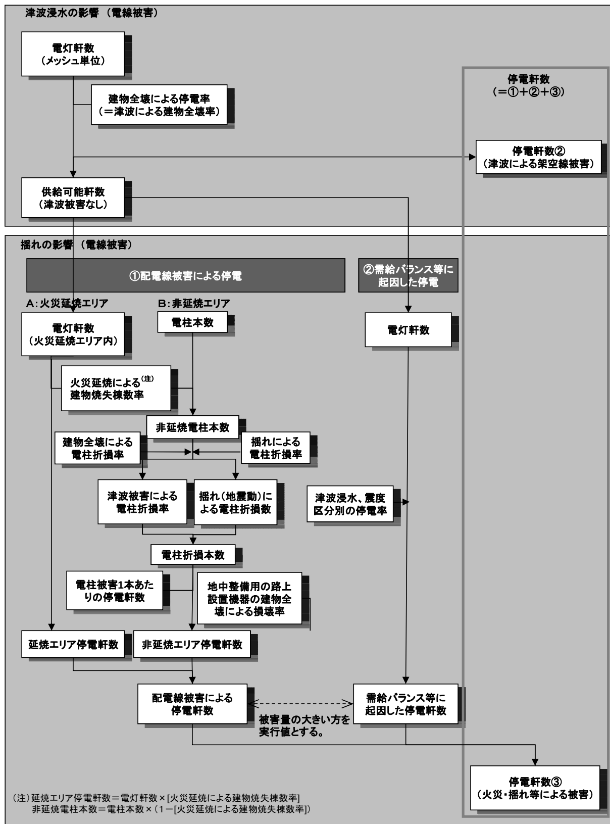
図4.3.1 停電軒数の算出フロー
