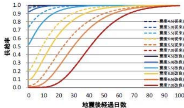
図 4.1.4 計測震度による供給率曲線の予測モデル（能島ら(2012) [5] ：上水道）
